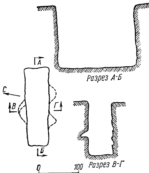
Рис. 3. Могила № 1419, вырубленная в скале. Раскопки К. К. Косцюшко-Валюжинича. Расчистка и обмеры 1975 г.
