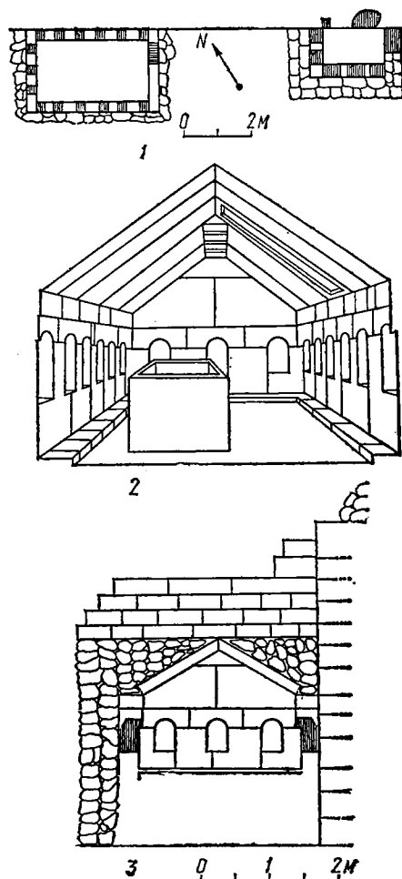
Рис. 12. Пристенные склепы № 1013, 1014. По Г. Д. Белову:
